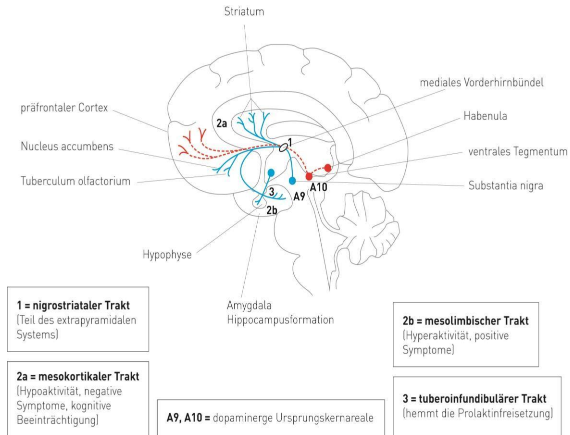
Abb. 3: Dopaminerge Systeme
